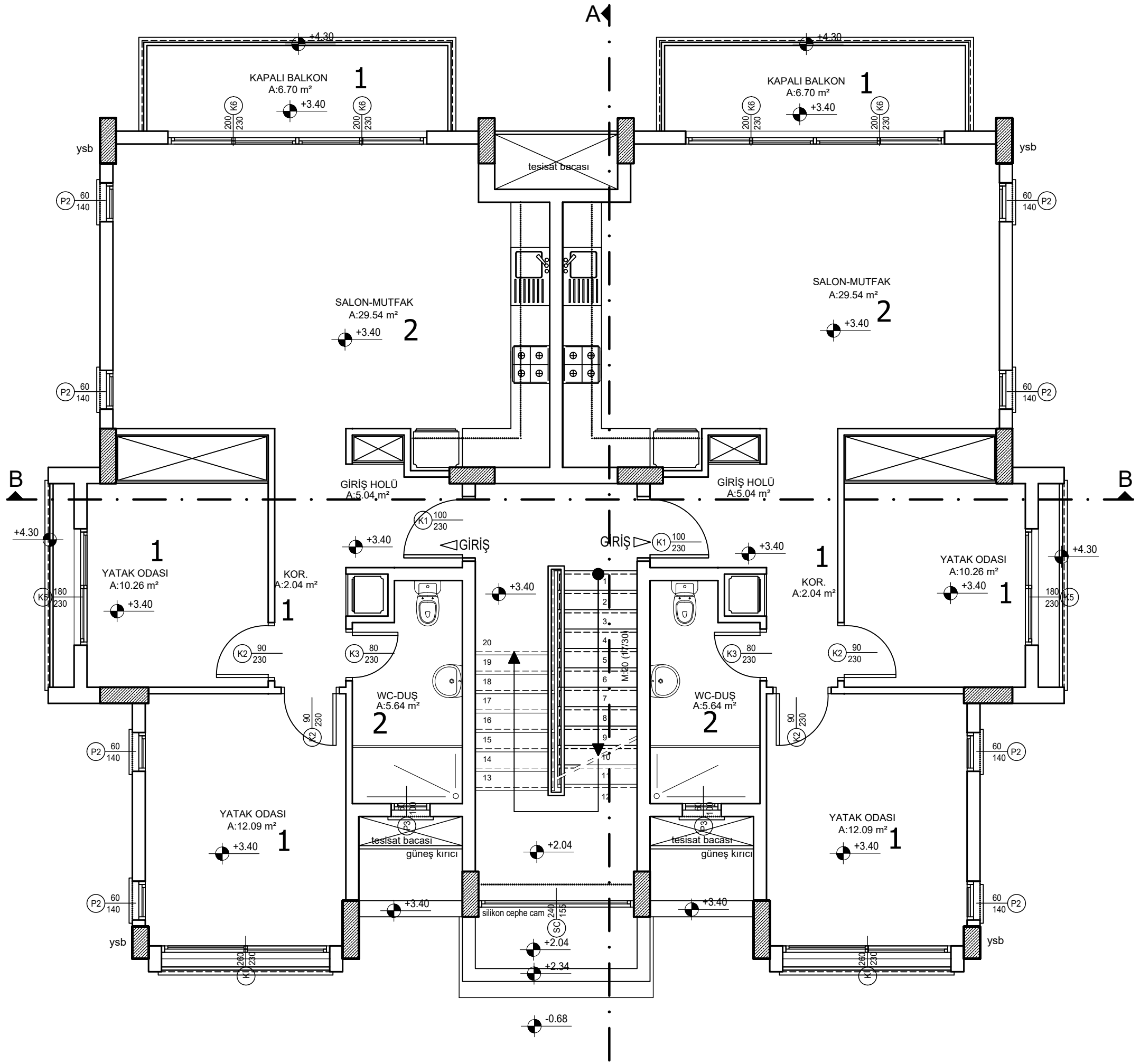
1. KAT PLANI ÖLÇEK: 1/50
